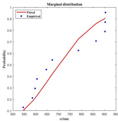
شکل ۳: توزیع حاشیه ای و توزیع نرمال متغیر جرم سرقت
