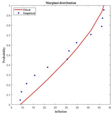
شکل ۲: توزیع حاشیه ای و توزیع نرمال متغیر تورم
