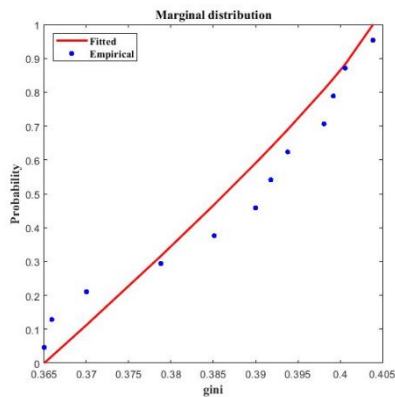
شکل ۴: توزیع حاشیه ای و توزیع نرمال متغیر ضریب جینی
