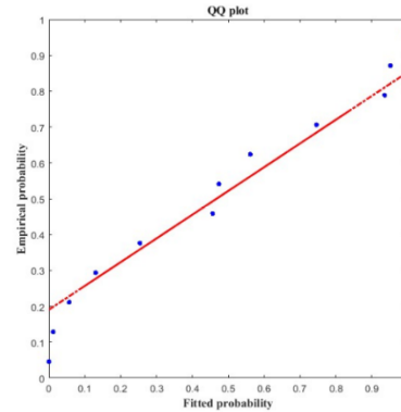
شکل ۲: توزیع حاشیه ای و توزیع نرمال متغیر تورم
