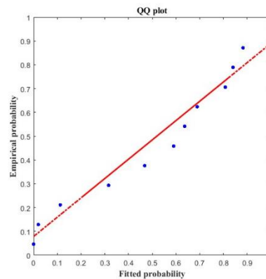
شکل ۴: توزیع حاشیه ای و توزیع نرمال متغیر ضریب جینی
